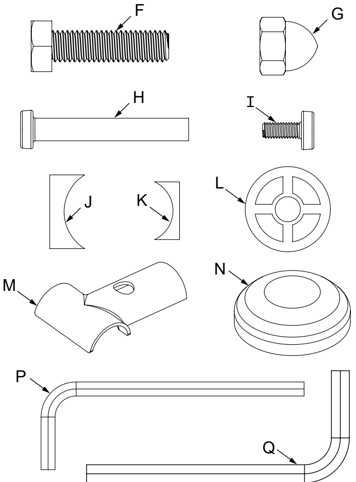
Paquete de hardware
